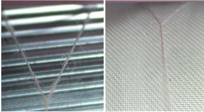
Triángulo de torcido en el proceso normal de hilado Siro
